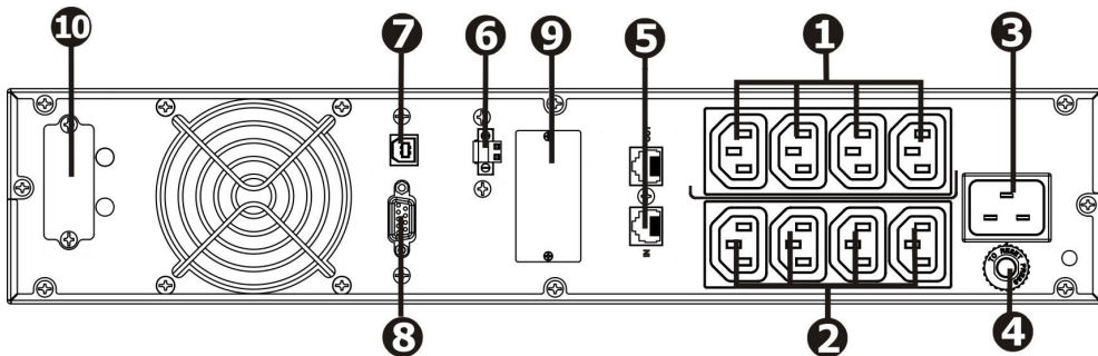
Рисунок 5 - Задняя панель ИБП АТС 2000 R-X, АТС 2000 R-BX, АТС 2000 R-BX (S), АТС 2000 R-BX (LS)
