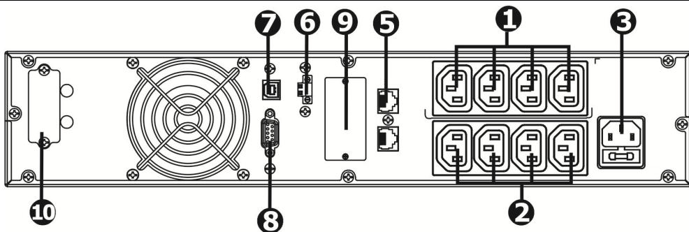
Рисунок 4 - Задняя панель ИБП АТС 1000 R-X, АТС 1000 R-BX, АТС 1000 R-BX (S), АТС 1000 R-BX (LS), АТС 1500 R-X, АТС 1500 R-BX, АТС 1500 R-BX (S)
