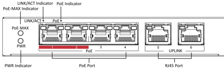
Рисунок 1.3 Передняя панель устройства
