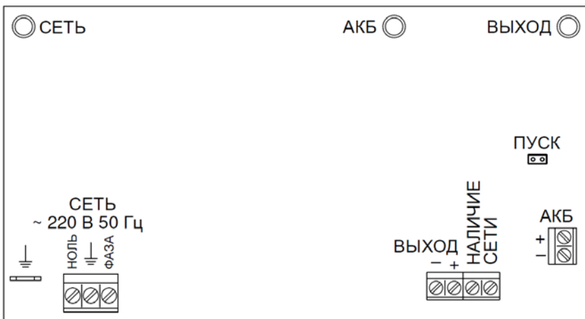
Рисунок 2 - общий вид платы
